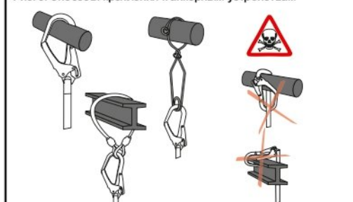
Рис. 5. Способы крепления к анкерным устройствам
