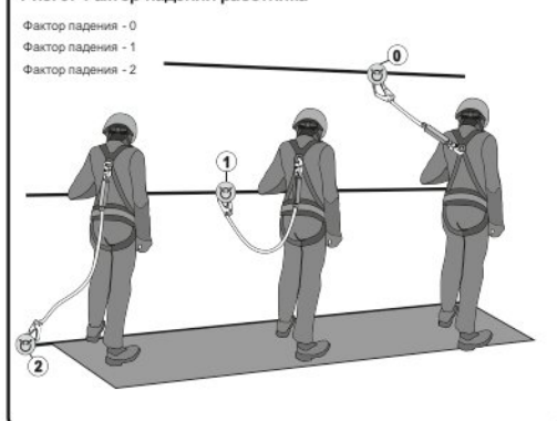
Рис. 11. Использование стропов без амортизатора
