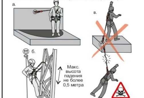
Рис. 11. Использование стропов без амортизатора
