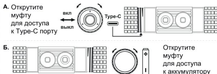
Рис. 7. СПОСОБ ДОСТУПА К АККУМУЛЯТОРУ И TYPE-C ПОРТУ
