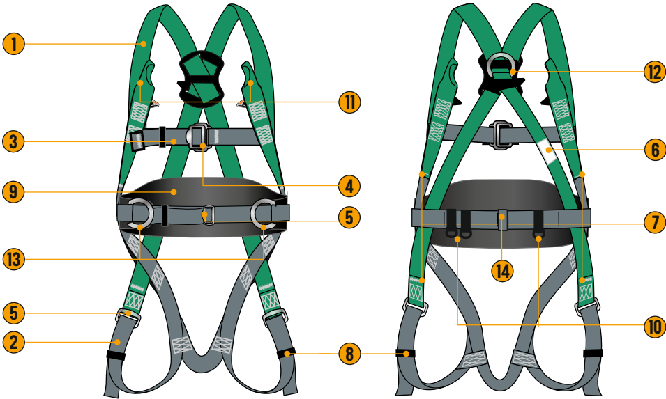
Рис. 2 Страховочная привязь LITE, арт. HS-05.
