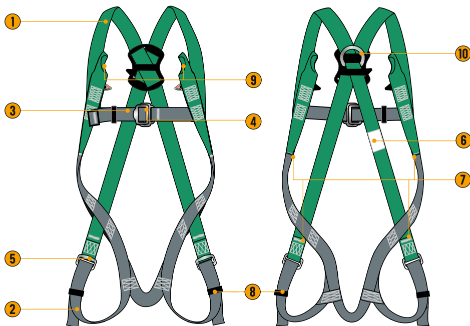
Рис. 1 Страховочная привязь LITE, арт. HS-03.
