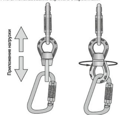
Рис. 2. Использование вертлюга с карабинами
