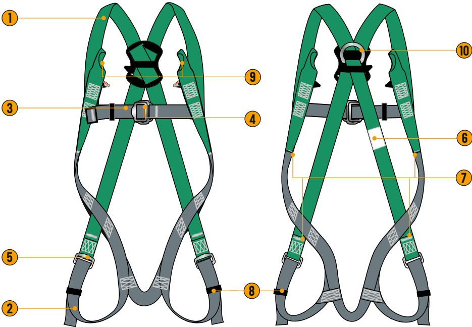
Рис. 2 Страховочная привязь LITE, арт. HS-03.
