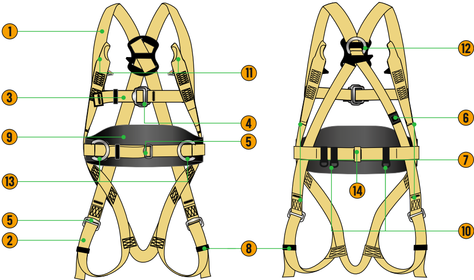
Рис. 2 Страховочная привязь LITE, арт. HS-05N.
