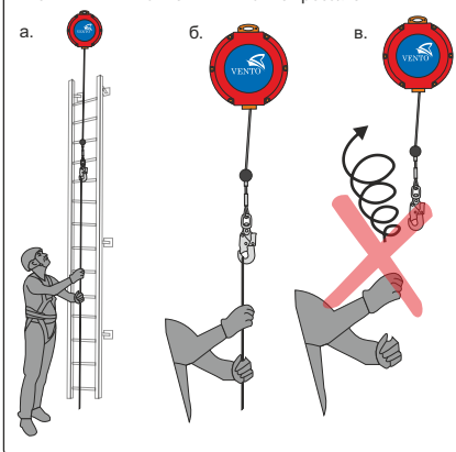
Рис. 12. Вытягивание и втягивание троса/ленты
