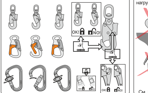
Рис. 9. Ограничения по использованию блокирующих устройств тягивающего типа НВ
