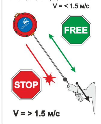
Рис. 13. Проверка перед использованием V < 1.5 м/с
