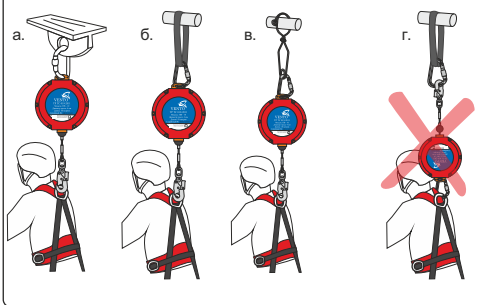
Рис. 6. Общие принципы использования карабинов
