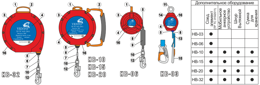
Рис. 3. Составные части блокирующих инерционных устройств тягивающего типа «НВ» (ООО «ВЕНТО-2М» оставляет за собой право на внесение изменений в выпускаемую продукцию, не влекущих изменений эксплуатационных свойств)
