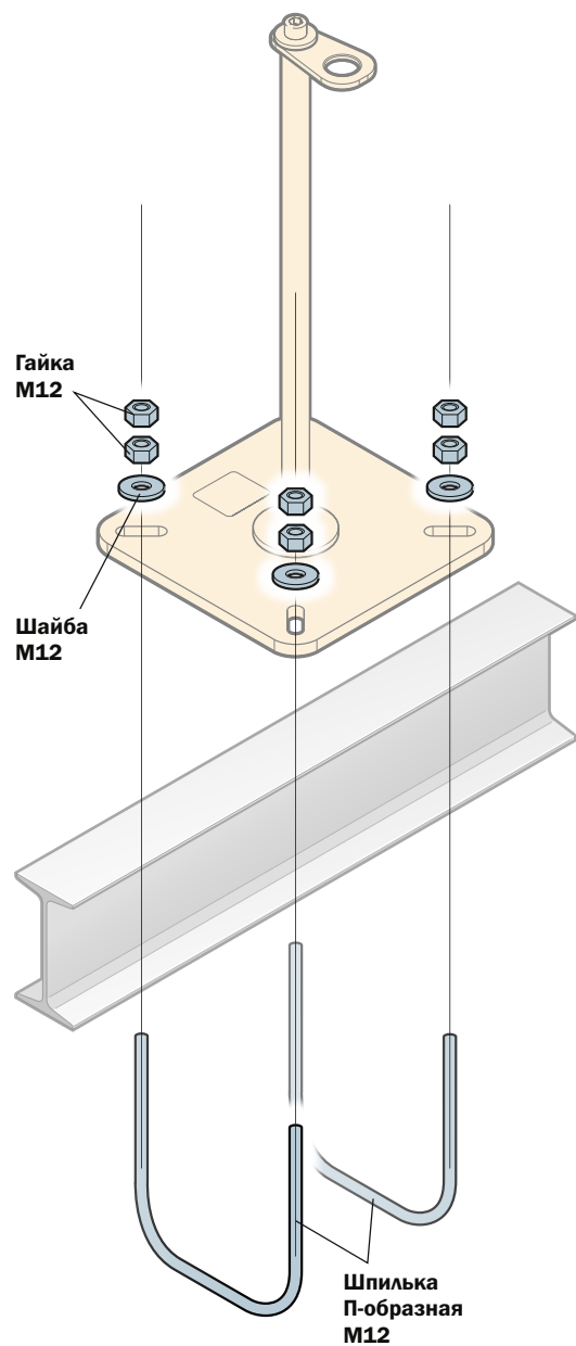
Рис. 5 Установка (монтаж) анкерных столбов.
